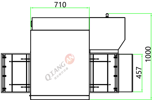
俯视图
