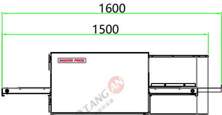
主视图
